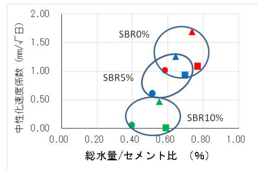
図-3 中性化速度係数
