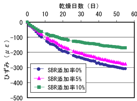
図-2 乾燥縮ひずみ
