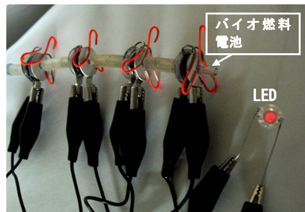
図1. バイオ燃料電池の発電の様子
