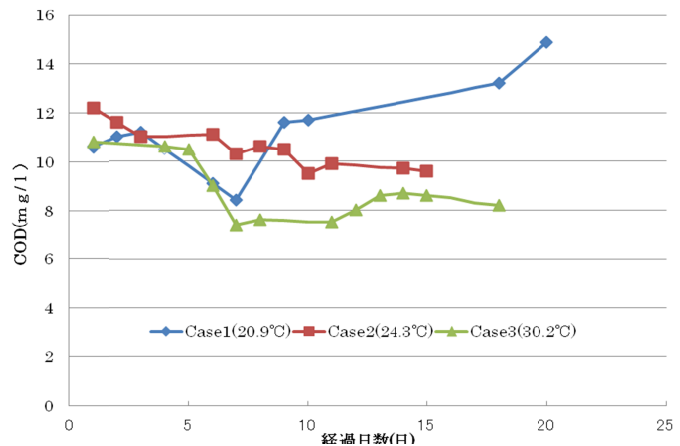
多孔質コンクリートブロックの COD の時系列変化
