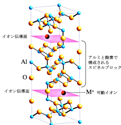
図1. βアルミナの基本格子
