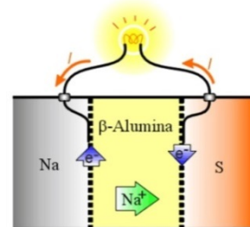
図2. NAS 電池の模式図
