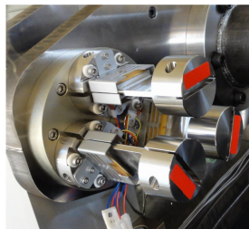
2 軸圧電アクチュエータ
