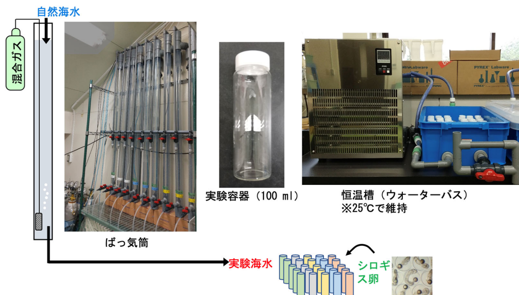
図1. 研究で使用した飼育実験システムの概要図（海生研提供）
