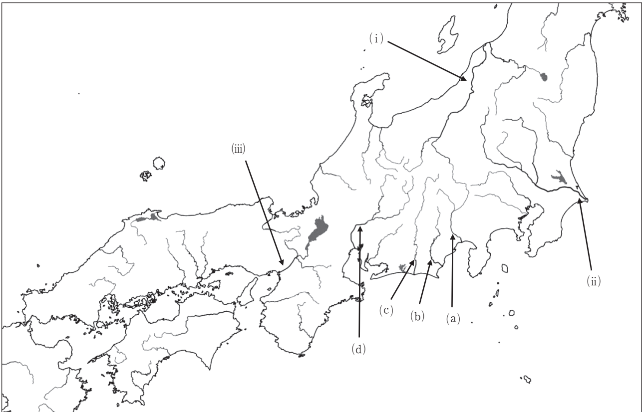
図1：本州の主要河川図(地理院地図をもとに作製)
