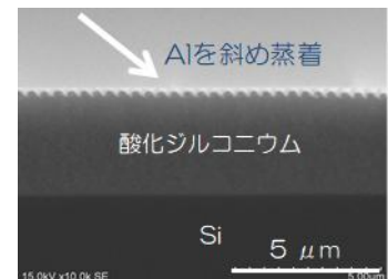
図2 作製したワイヤグリッド偏光子。
